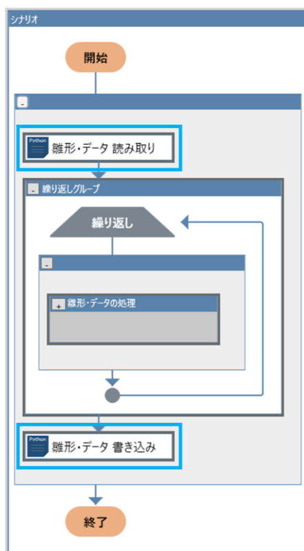
図 98-2 「雛形・データ 読み取り」ライブラリと「雛形・データ 書き込み」ライブラリのシナリオ例
