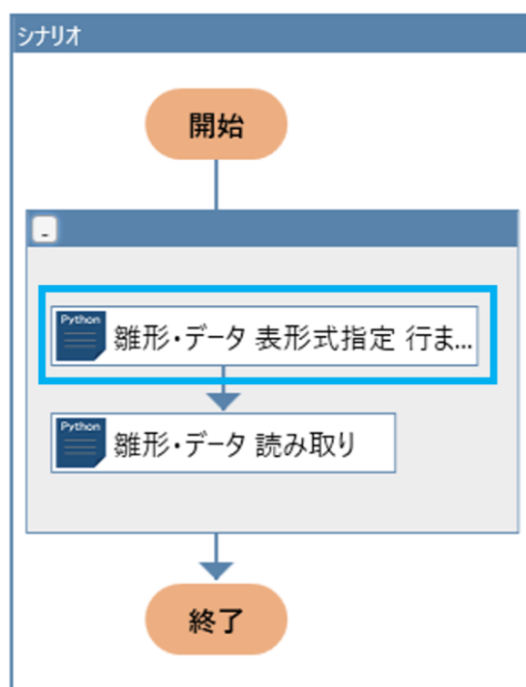
図 98-1 雛形・データ 表形式指定 行または列の挿入のシナリオ例
